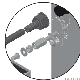
DETALLE BB
