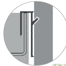
DETALLE HH
