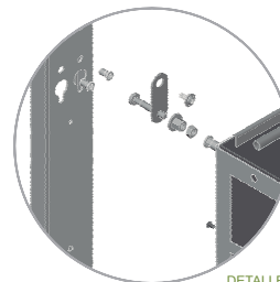
DETALLE BB
